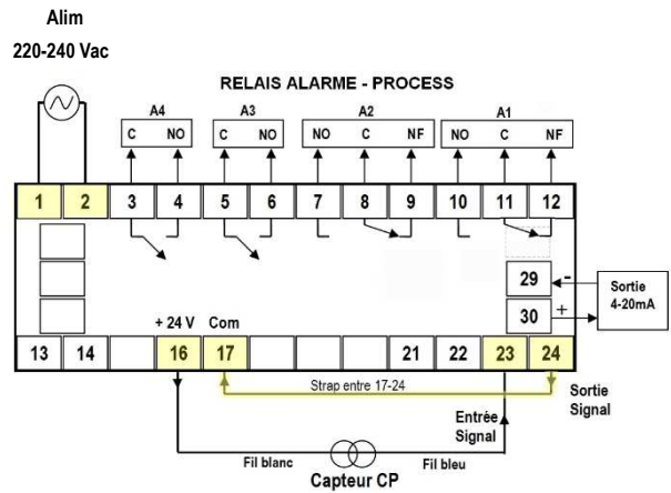
Fig. 1 – Raccordements du panneau arrière
